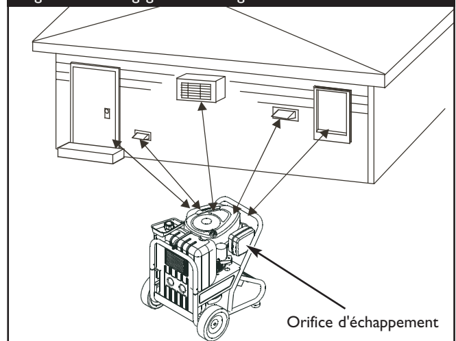
Figure 20 — Dégagement de la génératrice
